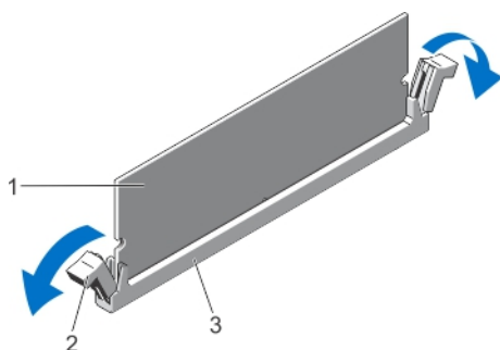
Ilustración 14. Expulsión del módulo de memoria
