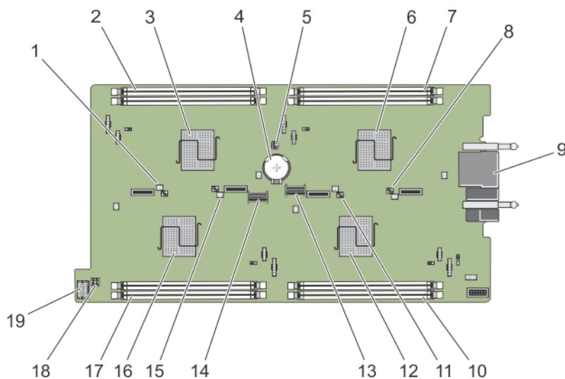
Ilustración 29. Conectores de la placa base
