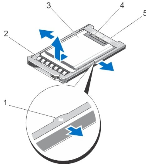
Ilustración 22. Extracción e instalación de una unidad SSD de 1,8 pulgadas en un portaunidades de SSD
