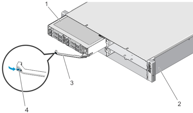
Ilustración 8. Extracción e instalación de un sled
