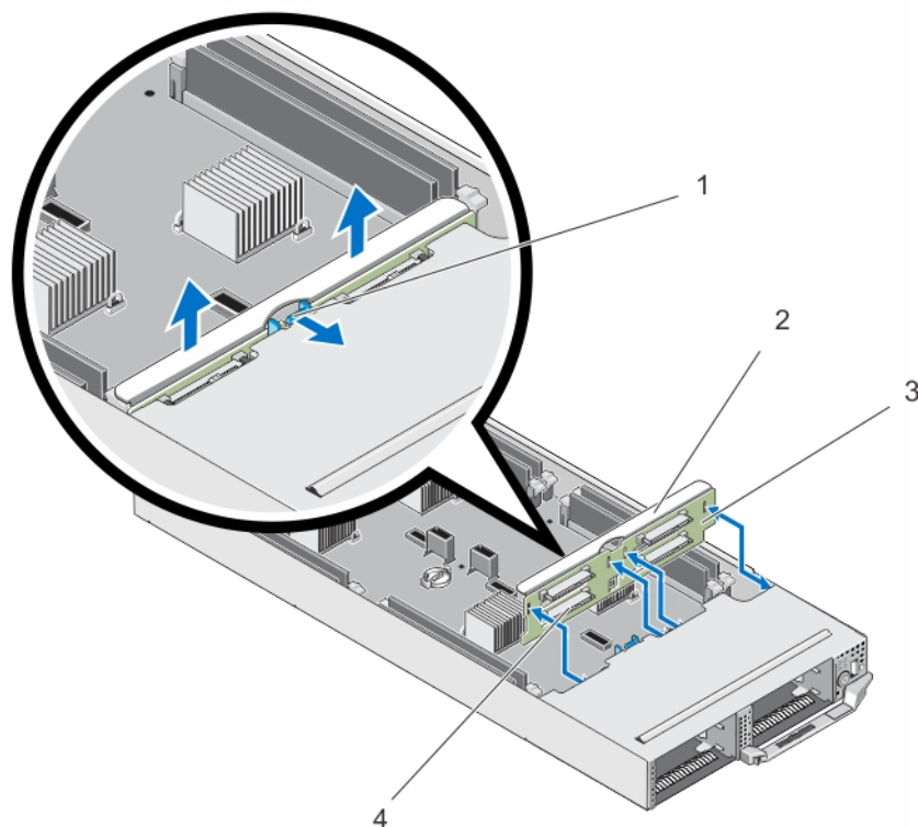
Ilustración 23. Extracción e instalación del plano posterior de la unidad de disco duro/SSD
