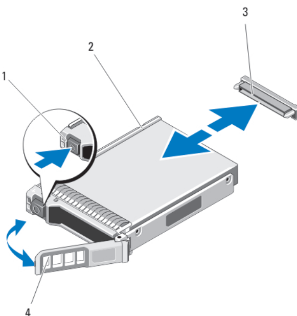
Ilustración 19. Extracción e instalación de la unidad de disco duro/SSD de 2,5 pulgadas
