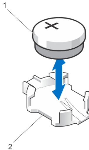
Ilustración 26. Sustitución de la batería del sistema
