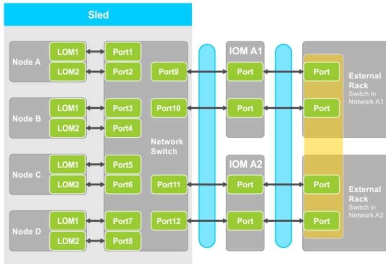
Ilustración 5. Configuración estándar
