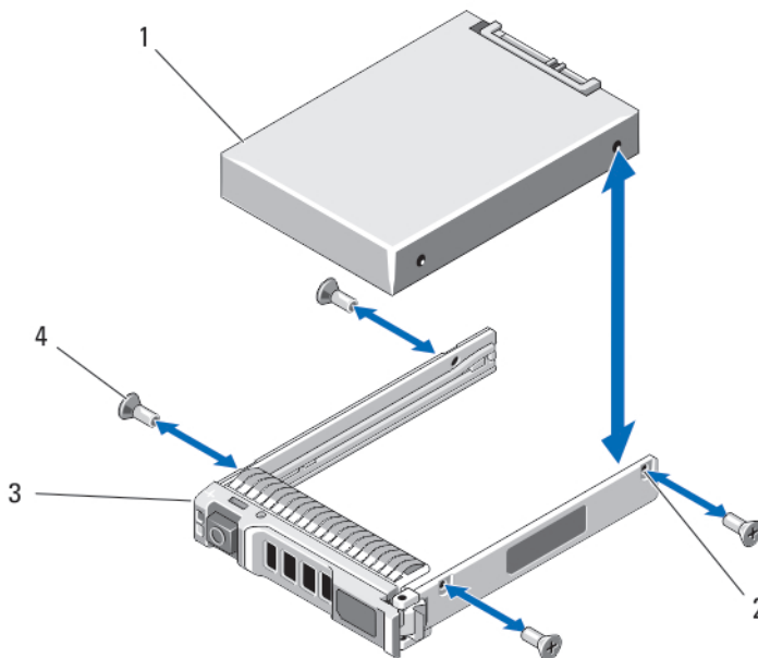
Ilustración 21. Extracción e instalación de una unidad de disco duro/SSD de 2,5 pulgadas del portaunidades de la unidad de disco duro/SSD
