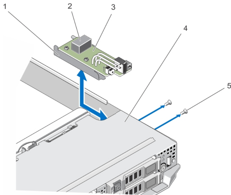
Ilustración 28. Extracción e instalación del panel de control
