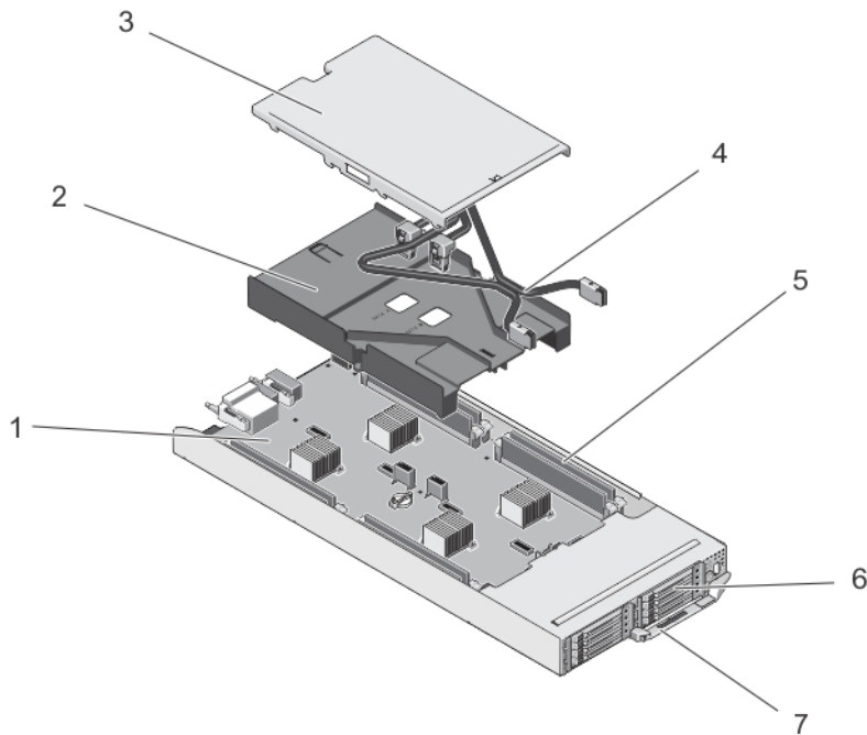
Ilustración 10. Interior del sled: sistema de SSD de 1,8 pulgadas
