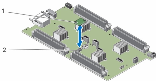
Ilustración 25. Colocación de un ERM
